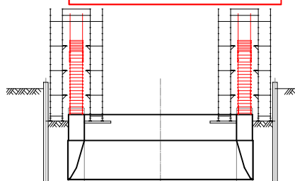
①鉄筋を組み立てます
