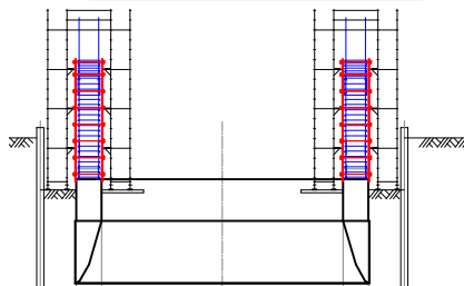
②型枠を組み立てます
