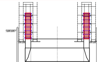
③型枠内にコンクリートを流し込みます
