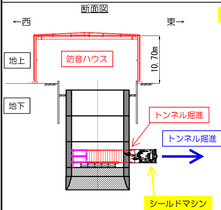
シールドマシン
