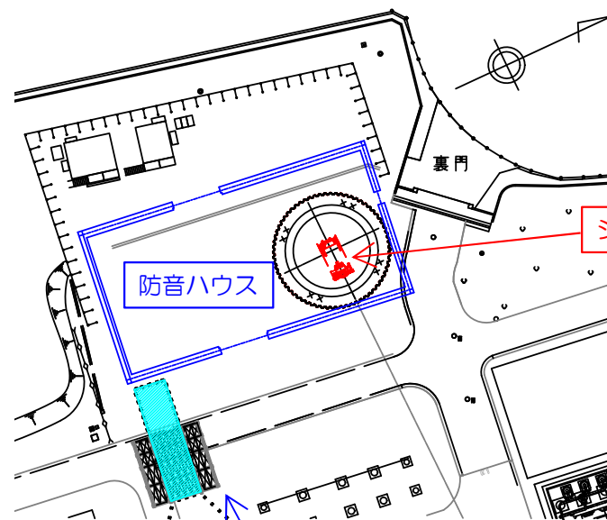
連系洞道掘削、土止め支保工
