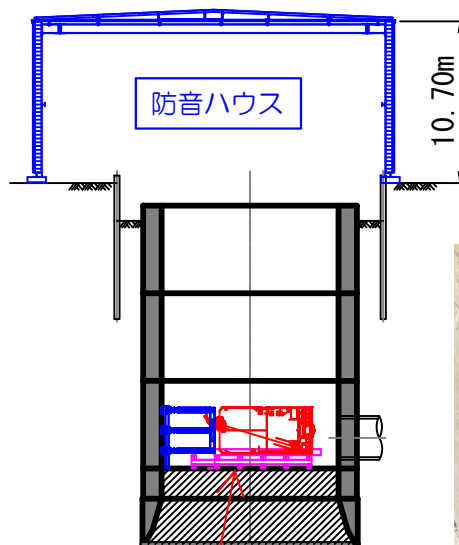
シールドマシン組立
