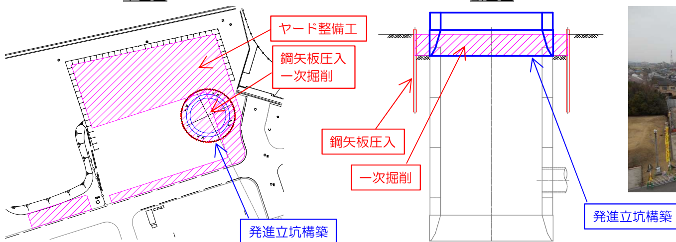
平面図
