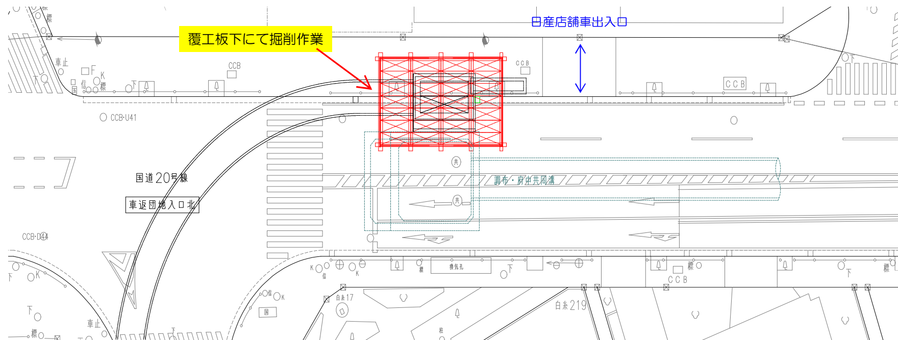
平面位置図
